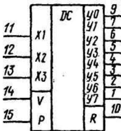
Условное графическое обозначение К155ИД13, КМ155ИД13
