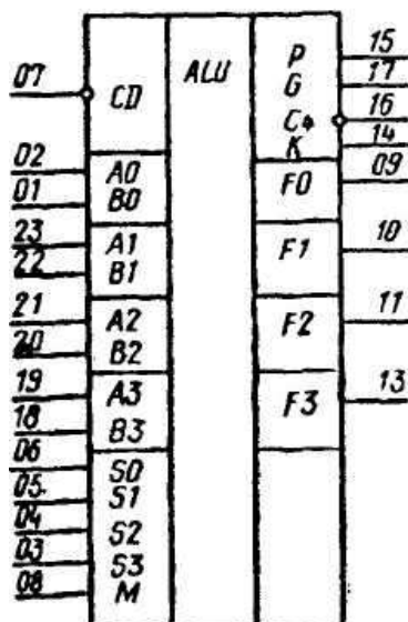
Условное графическое обозначение К155ИПЗ. КБ155ИПЗ-4
