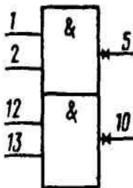
Условное графическое обозначение К155ЛИ5
