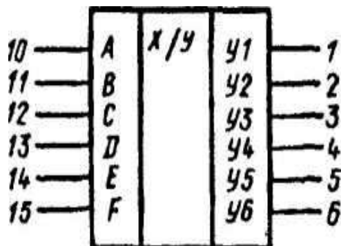
Условное графическое обозначение К155ПР7, КМ155ПР7
