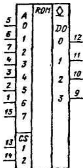
Условное графическое обозначение К155РЕ23
