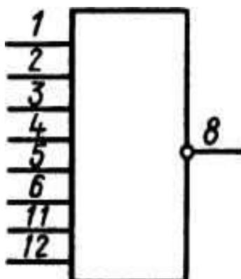
Условное графическое обозначение КР531ЛА2
