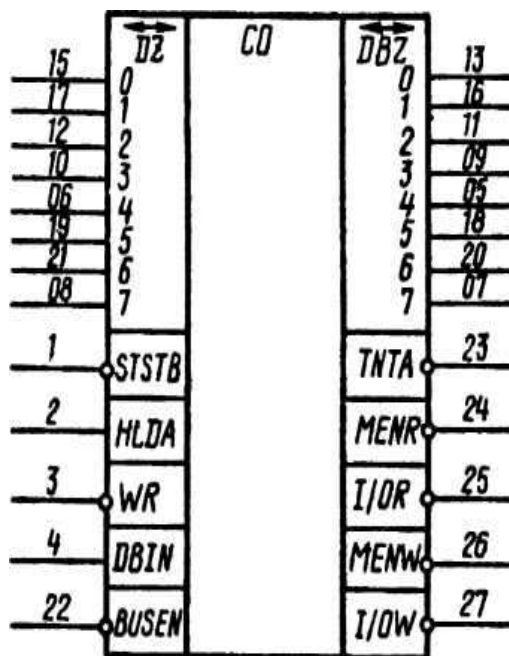
Условное графическое обозначение КР580ВК38
